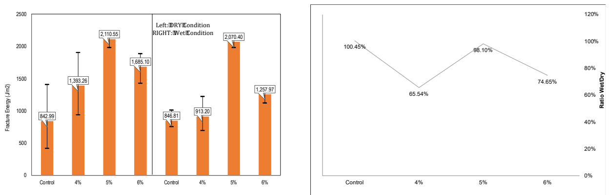
Gambar 8. Grafik Hasil Uji: (a) Energi fraktur dan (b) Rasio energi fraktur dalam kondisi basah dan kering
