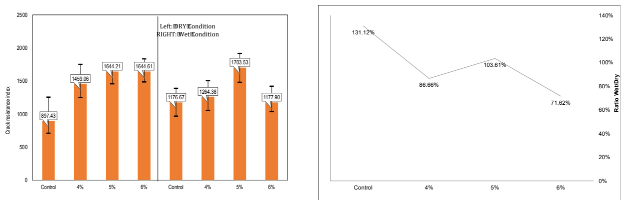
Gambar 9. Grafik Hasil Uji: (a) Crack resistance index (CRI) dan (b) Rasio CRI dalam kondisi basah dan kering
