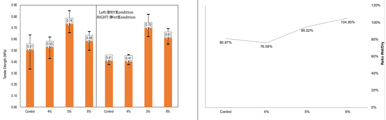
Gambar 7. Grafik Hasil Uji: (a) Kuat tarik dan (b) Rasio kuat tarik dalam kondisi basah dan kering
