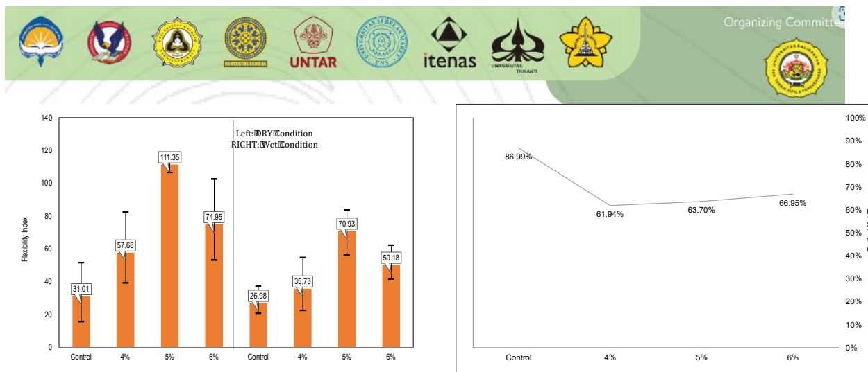
Gambar 10. Grafik Hasil Uji: (a) Flexibility Index (FI) dan (b) Rasio FI dalam kondisi basah dan kering
