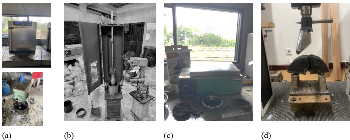
Gambar 5. Proses produksi sampel campuran aspal dengan langkah kerja (a) pemanasan di oven dan pencampuran di mixer, (b) kompaksi dengan mesin pemadat Marshall, (c) simulasi perendaman air di water bath , dan d) uji SCB di UTM
